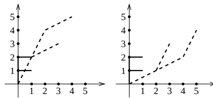
Abbildung 23.2. Orientierung am Buchstaben F: Das linke Bild zeigt F (durchgezogene Linien) und das Bild A(F) unter der Matrix A aus Beispiel 23.2 (gestrichelt). Das rechte Bild zeigt das entsprechende Resultat für die Matrix B .
