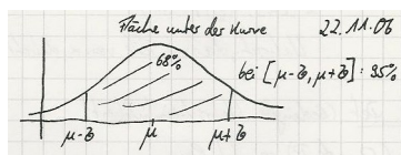
Abbildung 34.2. Die Normalverteilung.
