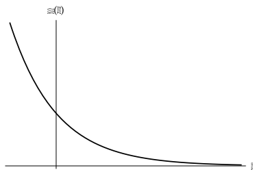
Abbildung 32.1. Radioaktiver Zerfall.
