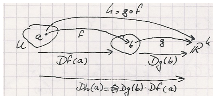
Abbildung 30.6. Die Kettenregel.
