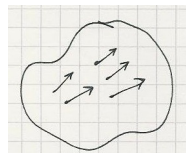
Abbildung 32.3. Ein Richtungsfeld.
