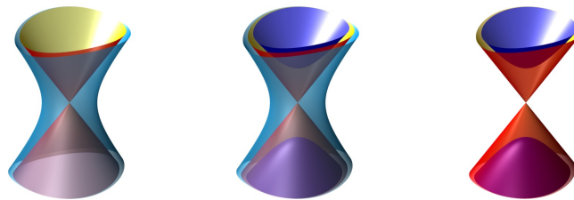
Abbildung 25.11. Hyperboloiden als Deformationen des Kegels: links der ein-, rechts der zweischalige und in der Mitte beide Deformationen gemeinsam.
