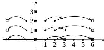
Abbildung 24.2. Die Operation der Matrix SAS^{-1} aus Beispiel 24.9, die Diagonalgestalt mit den Diagonaleinträgen 3 und 1 besitzt.
