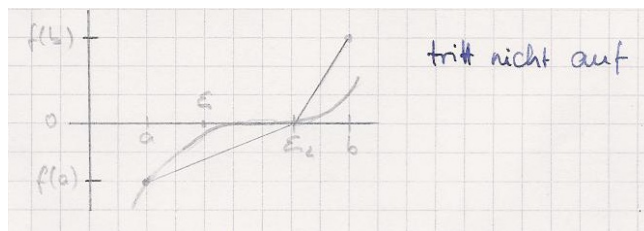
Abbildung 10.10. Konvexität erzwingt: höchstens eine Nullstelle.
