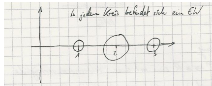
Abbildung 41.4. Drei Gerschgorin-Kreise.
