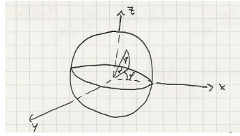
Abbildung 33.4. Kugelkoordinaten.
