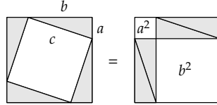
Abbildung 17.4. Dies zeigt: c^2 = a^2 + b^2 , da die vier Dreiecke gleich groß sind.
