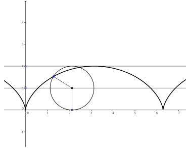
Abbildung 29.9. Die Zykloide.
