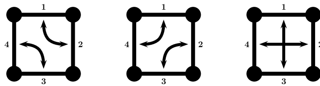
Abbildung 1. Die drei Paarungen \{(1, 2), (3, 4)\} , \{(1, 4), (2, 3)\} , \{(1, 3), (2, 4)\} der Menge \{1, 2, 3, 4\} .
