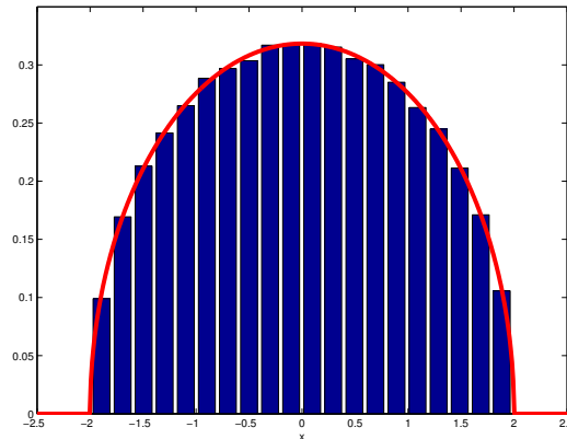
Abbildung 3. Vergleich der Halbkreisverteilung (rote Kurve) mit dem Histogramm (blau) der 4000 Eigenwerte einer gemäß der Verteilung (5) zufällig gewählten Gaußschen 4000 \times 4000 -Zufallsmatrix.
