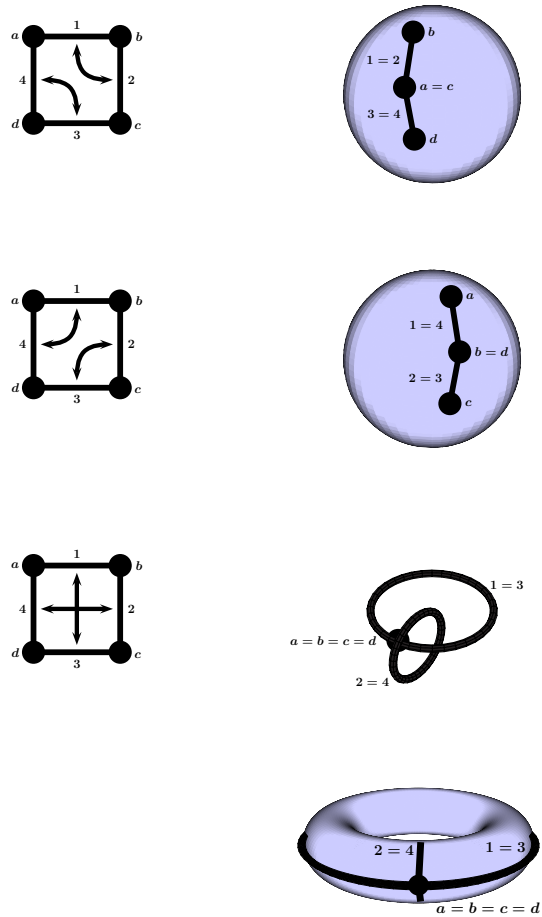
Abbildung 2. Graphen der drei Paarungen von 4 Elementen nach Identifikation der Kanten: die beiden ersten haben Geschlecht g = 0 und können ohne Kreuzungen auf einer Kugeloberfläche gemalt werden; die dritte Paarung kann ohne Kreuzung nur auf einem Torus gemalt werden und hat Geschlecht g = 1 ; man beachte auch, dass die beiden ersten Graphen drei Vertices haben, während der dritte nur einen Vertex besitzt, im Einklang mit Formel (2).
