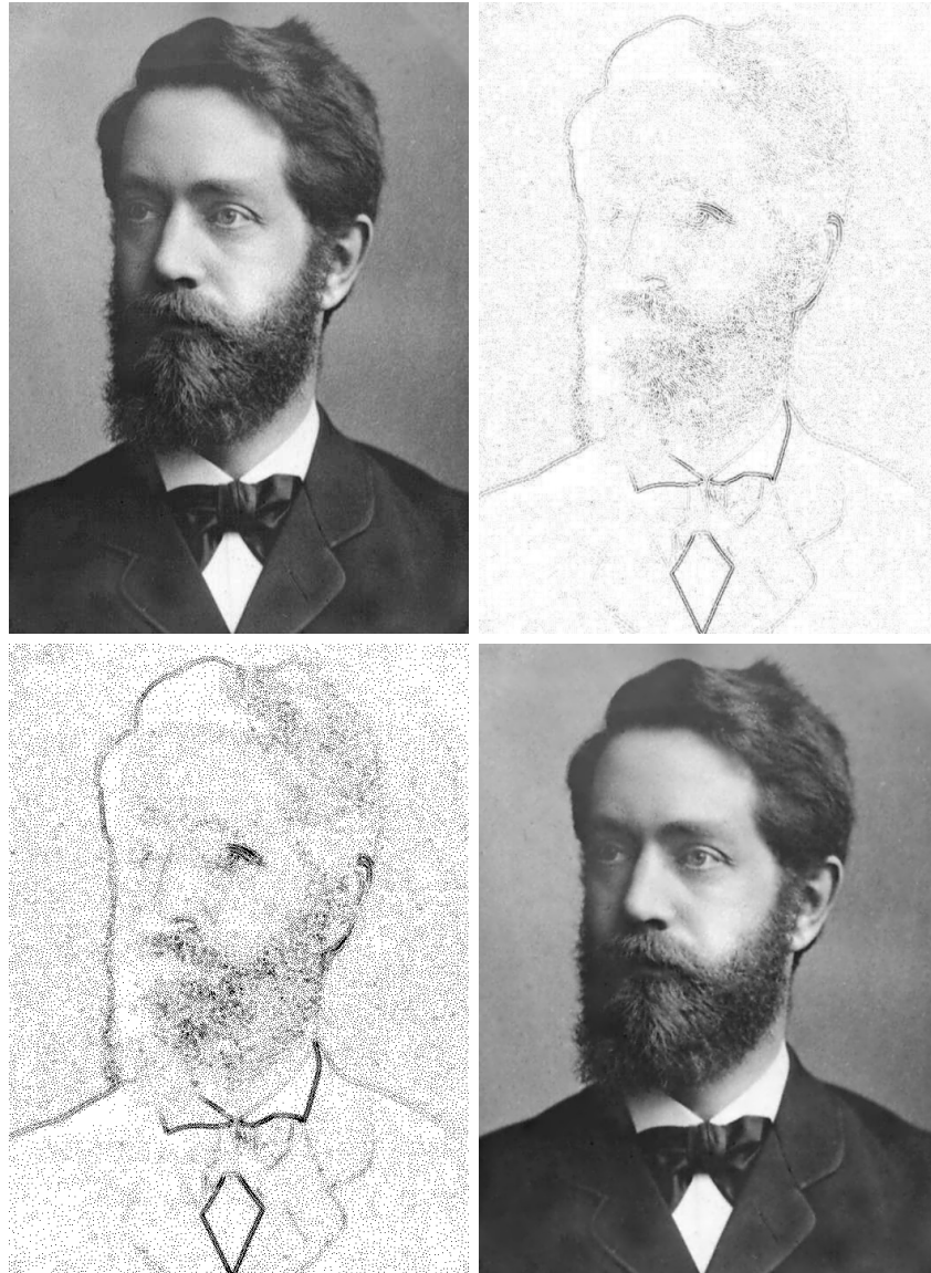
Abbildung 11: Oben links: Originalbild von Felix Klein, 512 \times 720 Pixel. Oben rechts: Betrag des Laplaceoperators. Dunkle Farben repräsentieren hier hohe Werte. Unten links: Ausgewählte Interpolationspunkte bei einer gewünschten Dichte von 10 %. Hierzu wurde elektrostatisches Halftoning verwendet. Unten rechts: Nach Interpolation mit der Laplacegleichung.
